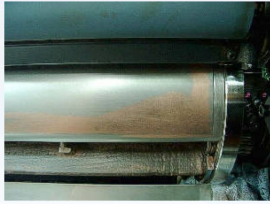
Reparaturbeispiel eines Korrosionsschadens an einem Gummizylinder
